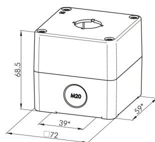
Maßskizze
